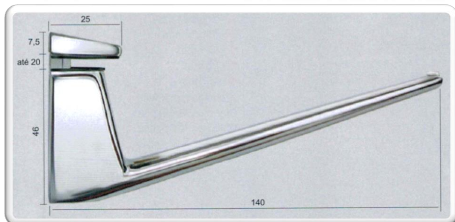
SUPORTE ÔMEGA VIDROS ATÉ 20 MM
