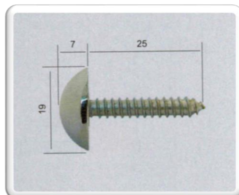
BOTÃO CABEÇA MACICA
